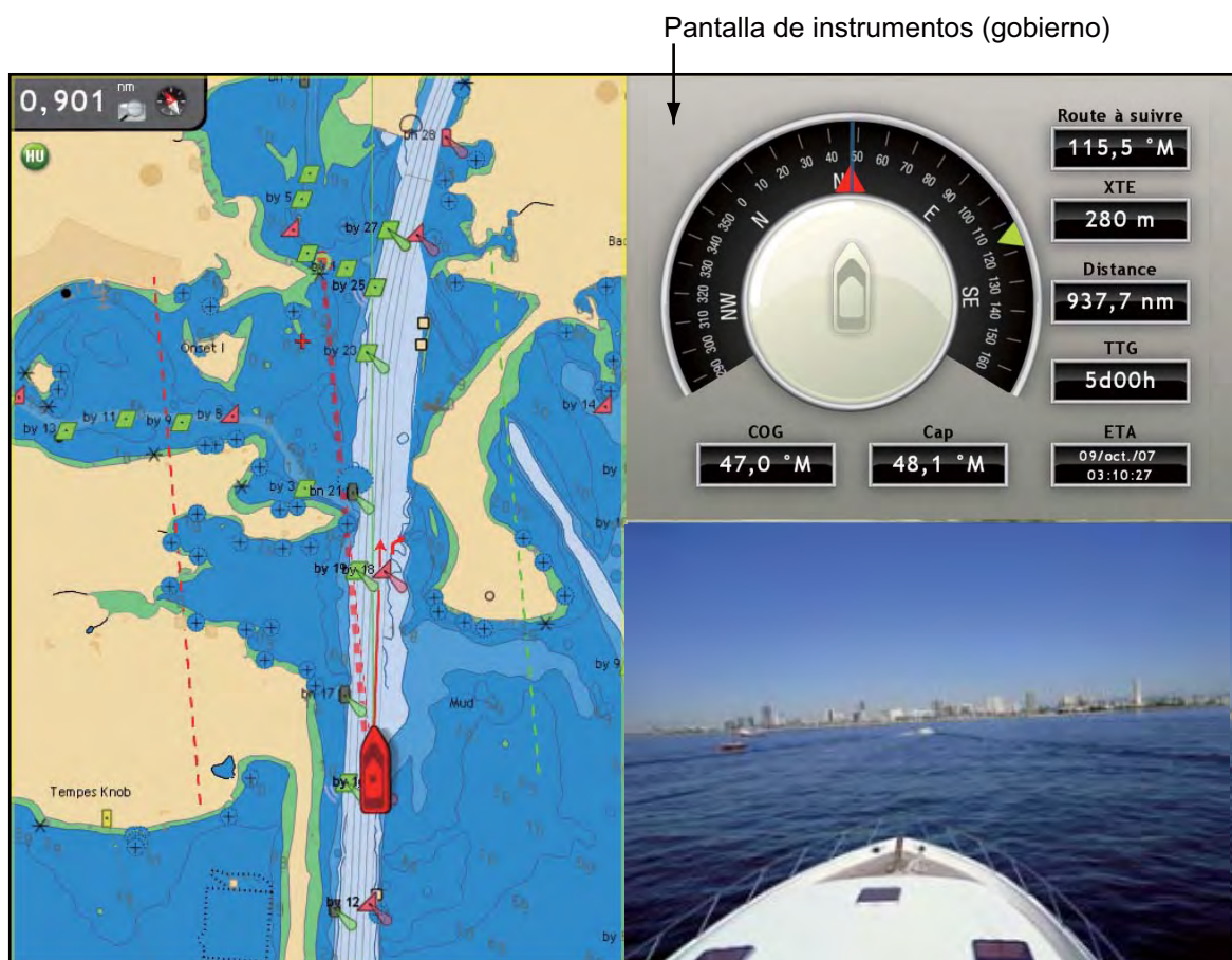
Pantalla de instrumentos (gobierno)
